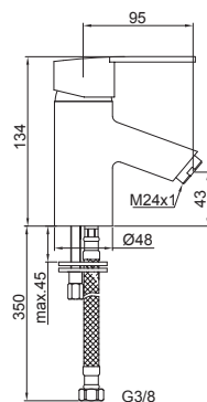
Monomando lavabo acabado cromo. Basin single-lever , chrome finish. Mitigeur lavabo , fini chromé.
