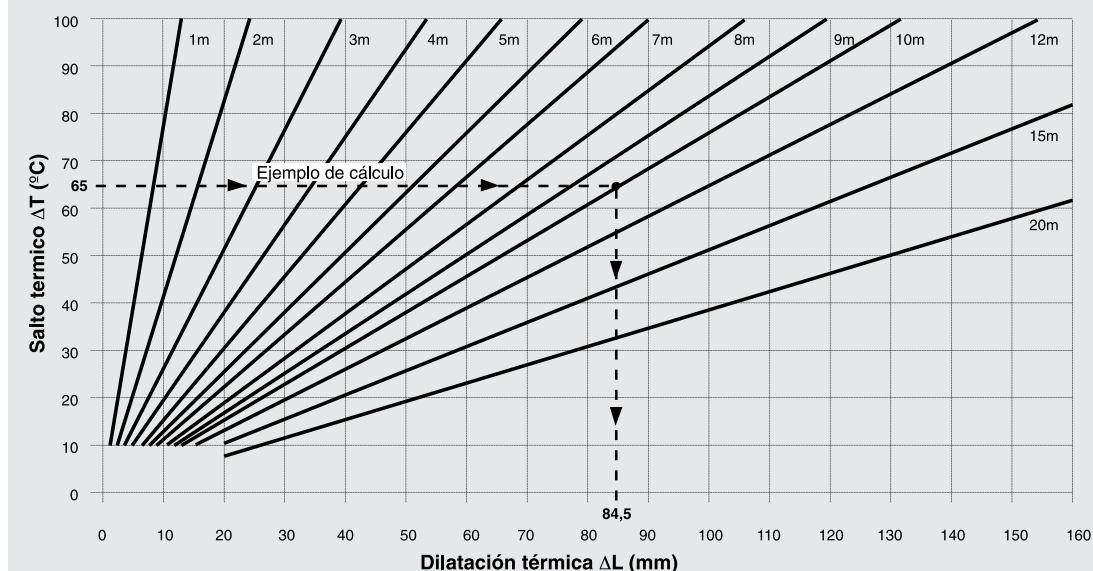
FIGURA 1.1 DIAGRAMA DE CÁLCULO DE DILATACIÓN TÉRMICA PB ELOTHERM
